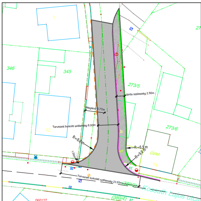
Ábra: 1.sz módosítás helyszínrajz, tervezett állapot (Forrás: Herend Város Önkormányzata)
