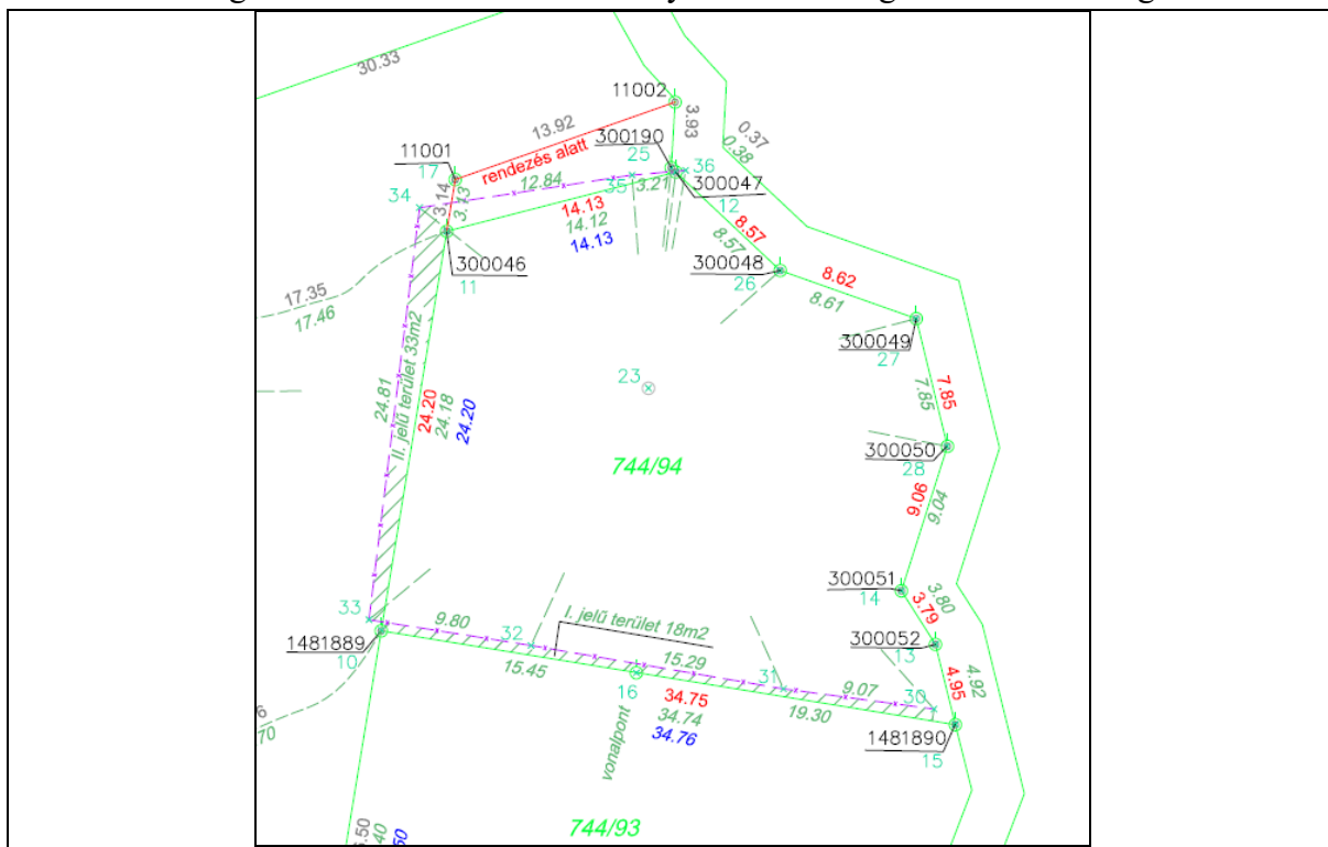
Ábra: Kitűzési vázlat, Németh László földmérő
